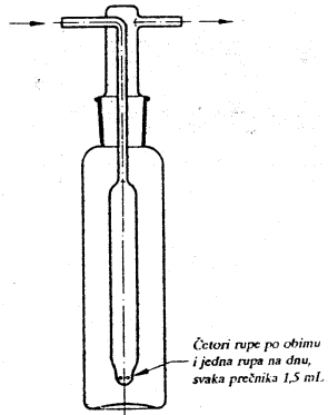
Apsorpciona boca (ispiralica) po Munku (Muenke) zapremine 50 mL.
